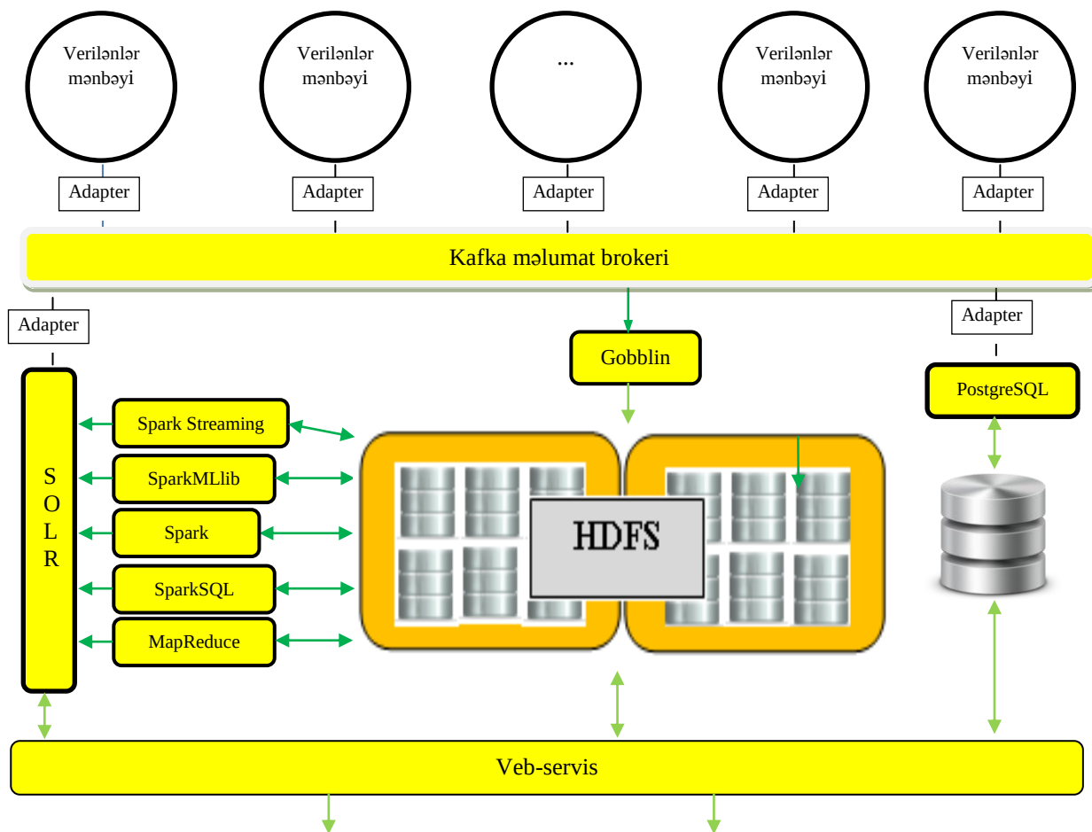
Şəkil 1. E-səhiyyə sistemi üçün konseptual Big Data arxitekturasının ümumi sxemi
