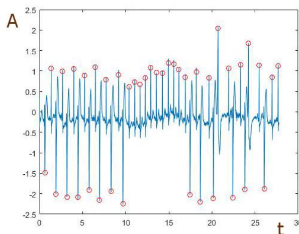
Şəkil 1. R-impulsların amplitudlarının müxtəlifliyi şəraitində R-R intervallının koordinatlarının müəyyənəndirilməsi.
