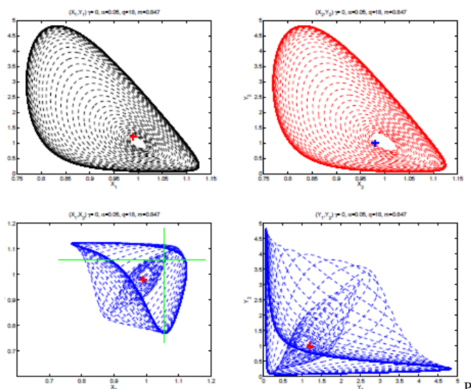
ис.2. Процесс репликации в отсутствие диффузии субстрата
