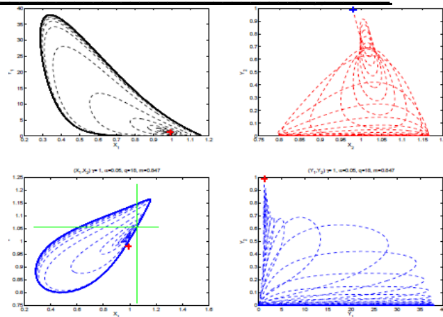
Рис.3. Малая диффузия субстрата приводит к вырождению одного из процессов репликации
